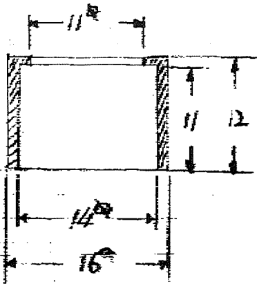
鋁殼 Bottom Alu. casting
